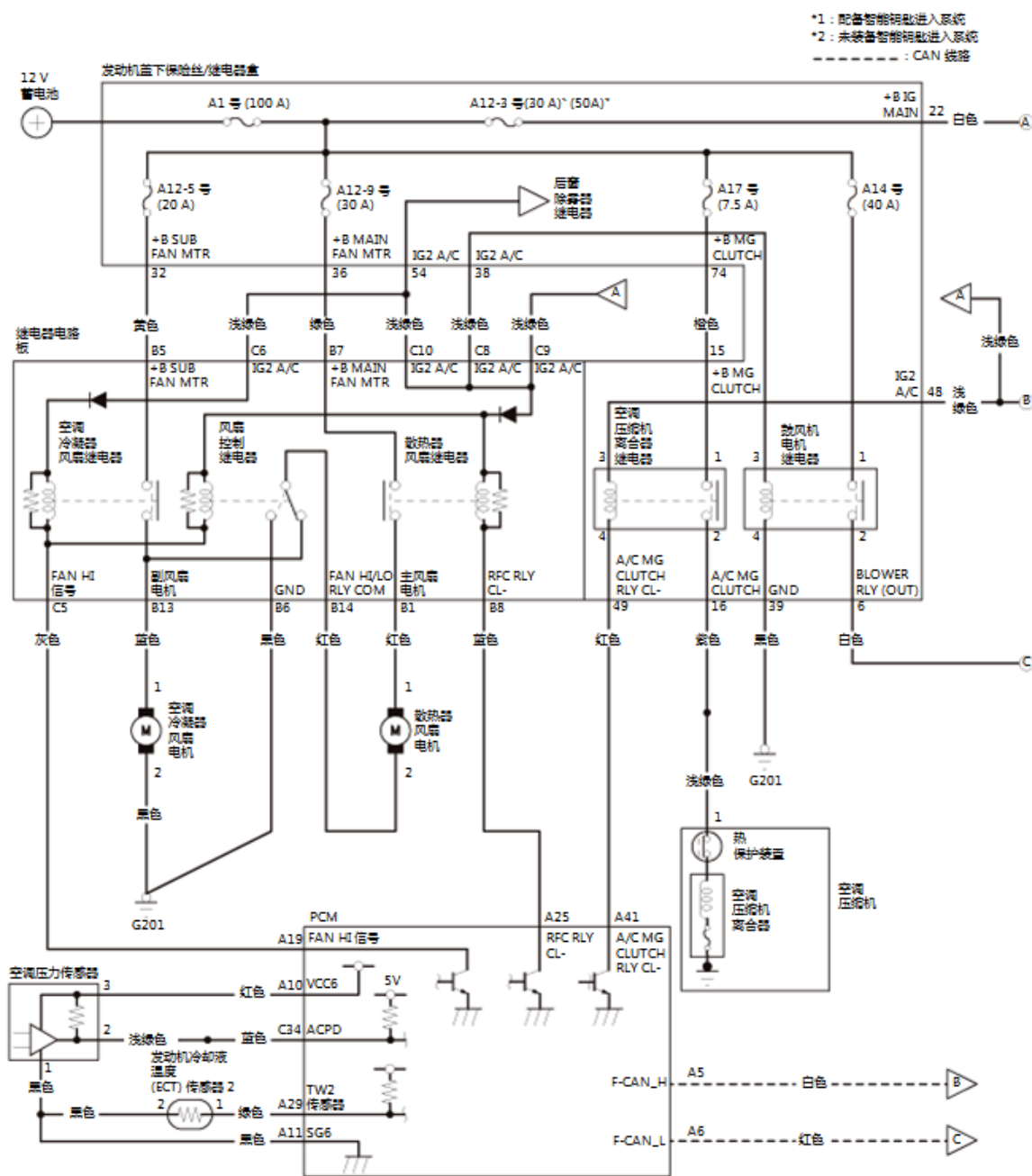
气温控制系统电路图
